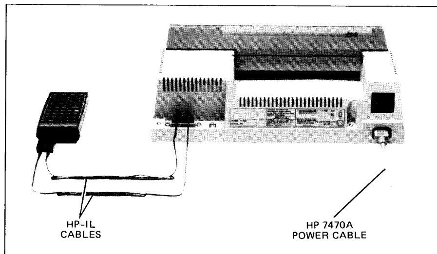
HP-IL Cable Connection
